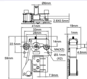
Raccordement direct surmicrorupteur
