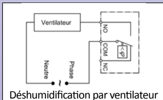
Déshumidification par ventilateur
